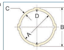
rura inklinometryczna
